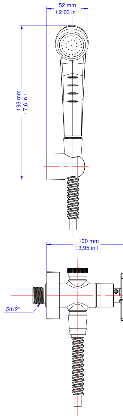
DUCHA HIG COM REGISTRO E DERIVAÇÃOC/ GATILHO DOCOL CITY - CHROME TOILET HANDSHOWER W/ VALVE AND OUTLET FOR TOILET TANK DOCOL CITY - CHROME DUCHA HIGIENICA CON LLAVE Y DERIVADOR DOCOL CITY - CHROME
